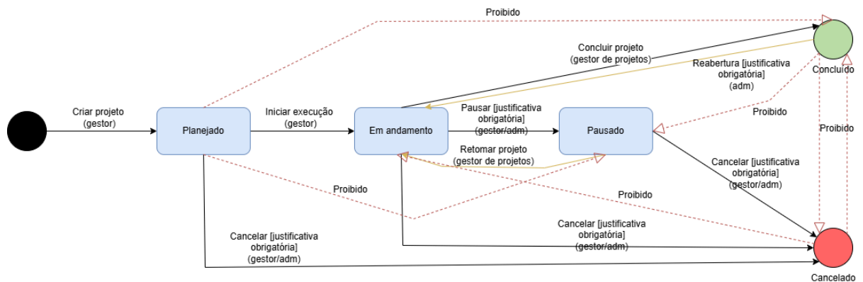
Figura 1 - Diagrama de estados do Projeto
