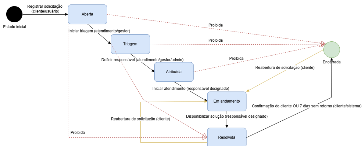
Figura 2 - Diagrama de estados da Solicitação
