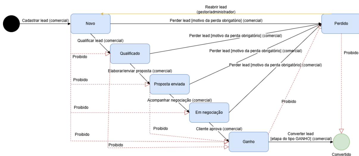
Figura 3 - Diagrama de estados do Lead
